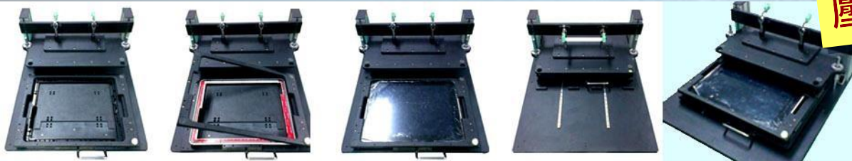
手動 / 壓合治具
