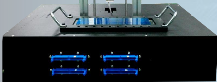
條板手動測試 / 線針治具
