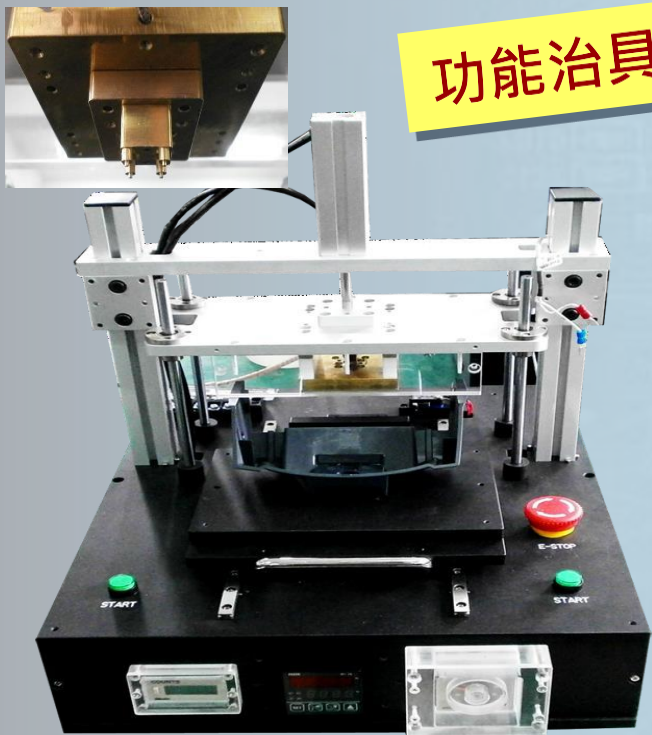
共用型 / 熱熔治具
